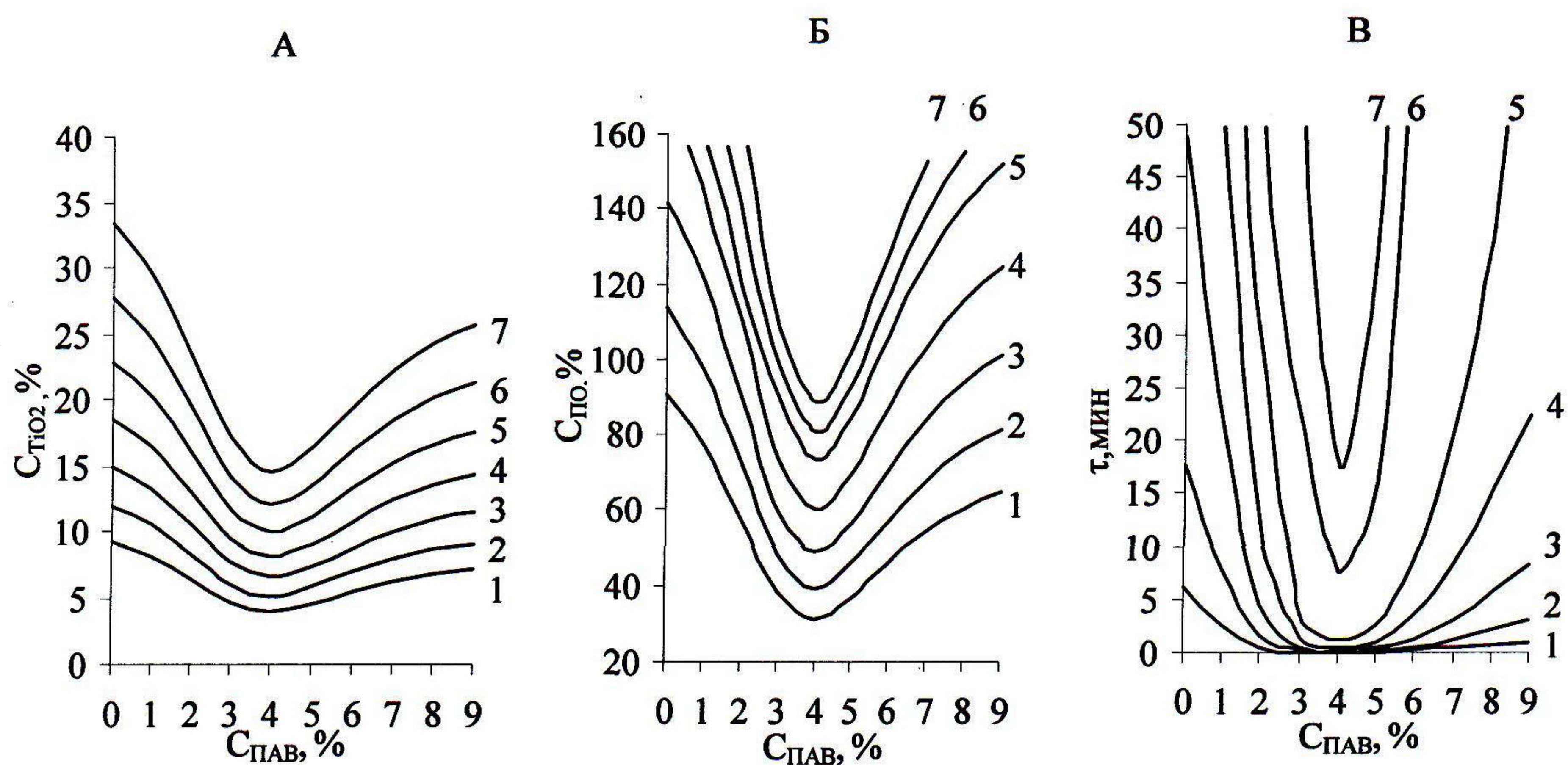
А, Б, В — системы с пентафталевым лаком, количество частиц: 1 — 2400; 2 — 2900; 3 — 3100; 4 — 3400; 5 — 3900; 6 — 4100; 7 — 4400
